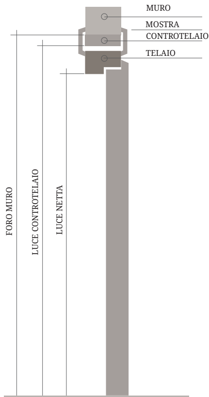
SEZ. VERTICALE
