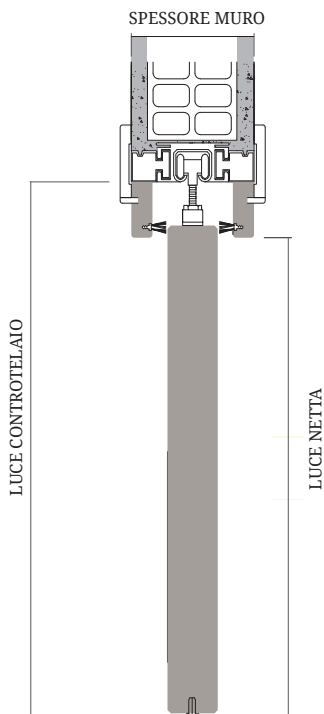
SEZ. VERTICALE
