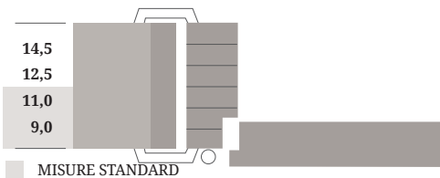
LARGHEZZA STIPITI
