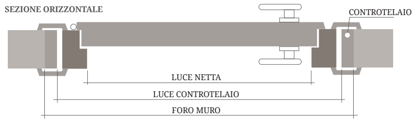
LARGHEZZA STIPITI
